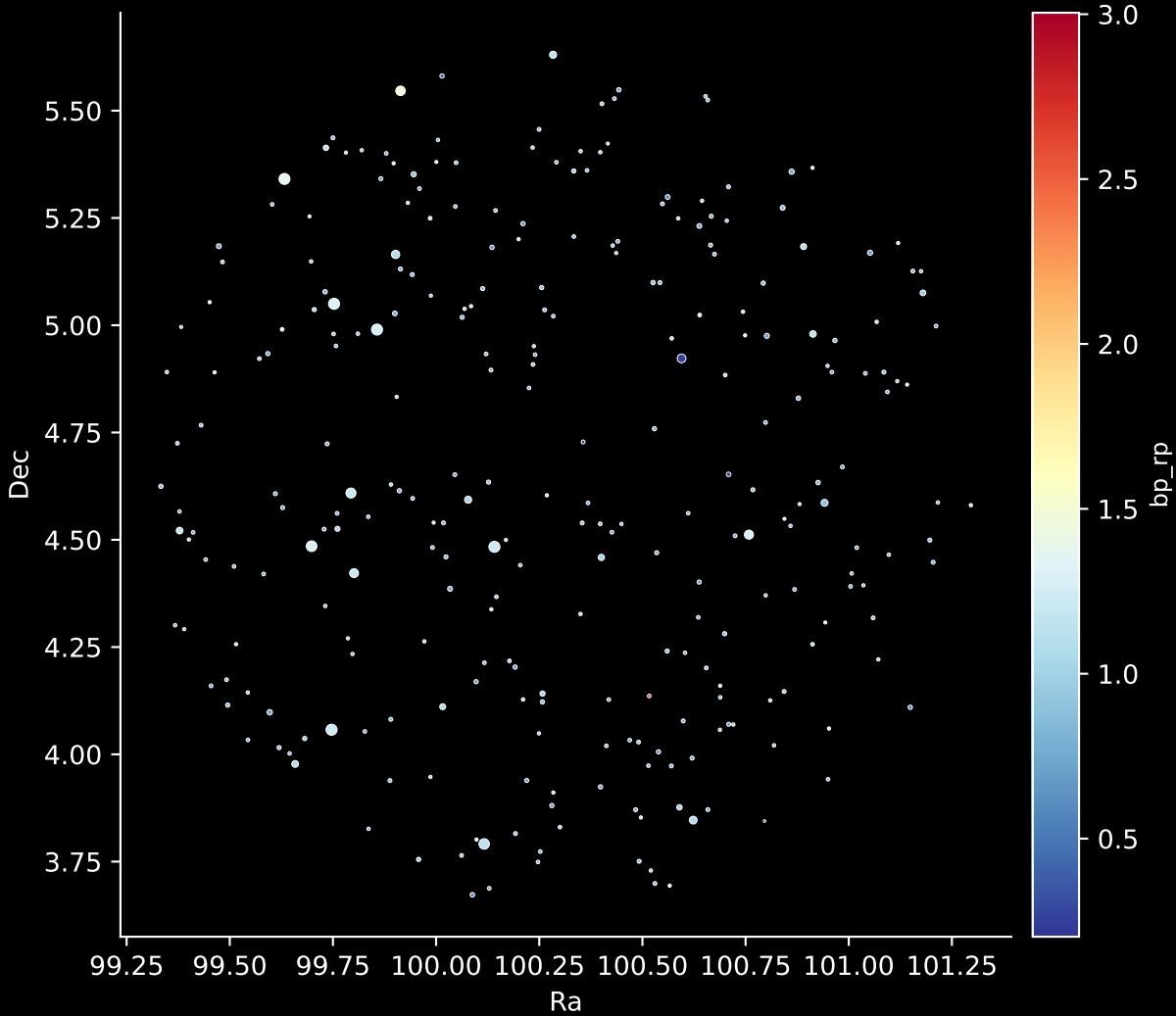
GALAH DR4 Field: [6882] Stars: 276
