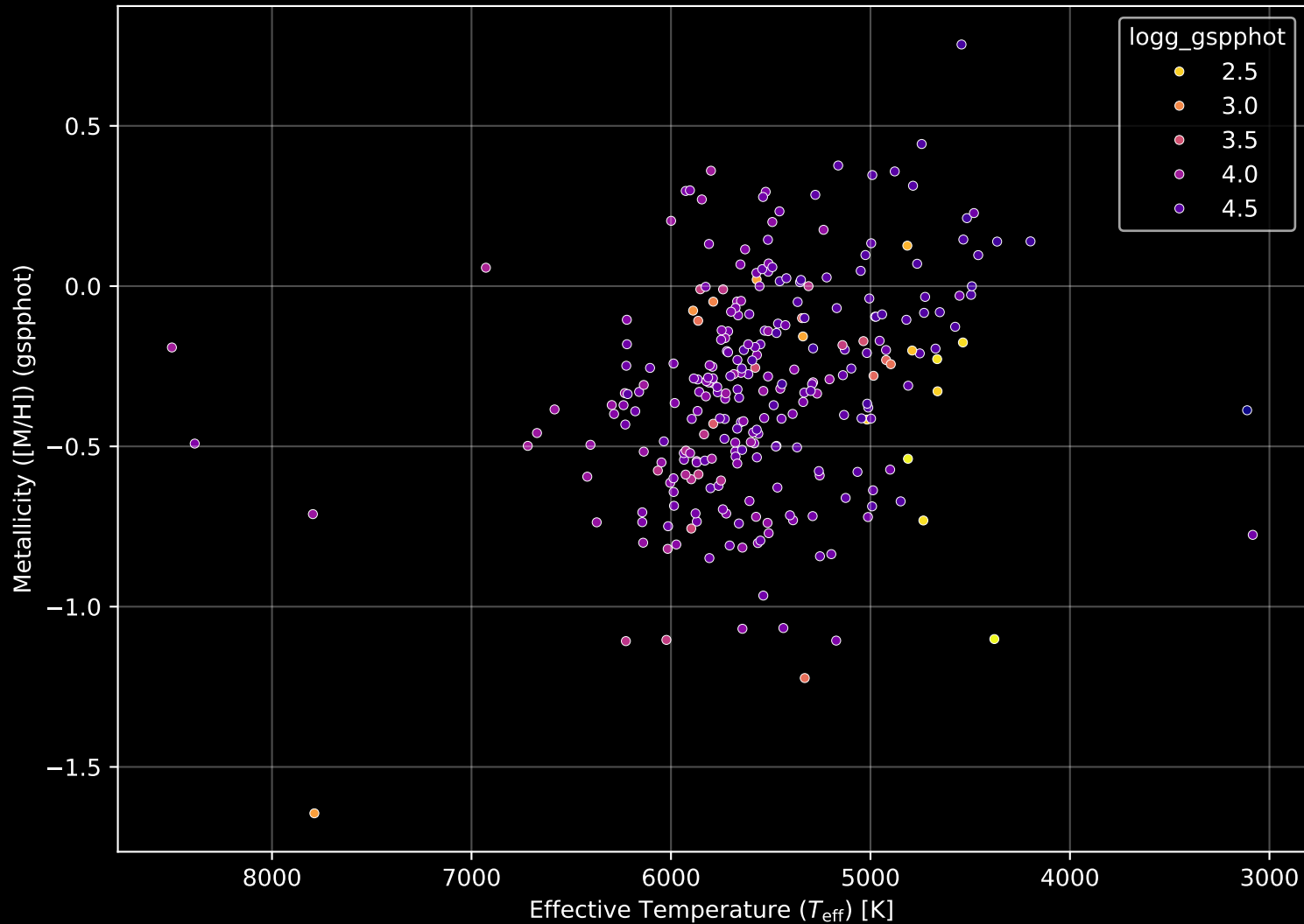
GALAH DR4 Field: [6882] Stellar Population Parameters (n= 276)
